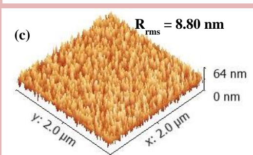
3D AFM images of TiO 2 thin films
