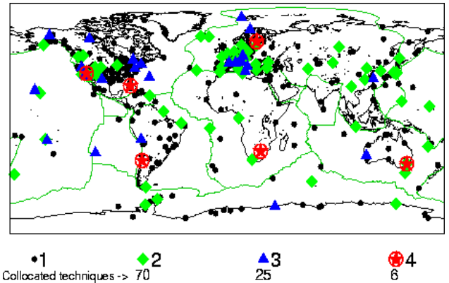
Figure 1. Le réseau primaire de l'ITRF2000
