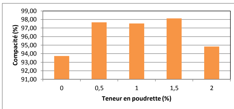
Figure 6. Compacités en fonction de la teneur en déchets « Mode B »
