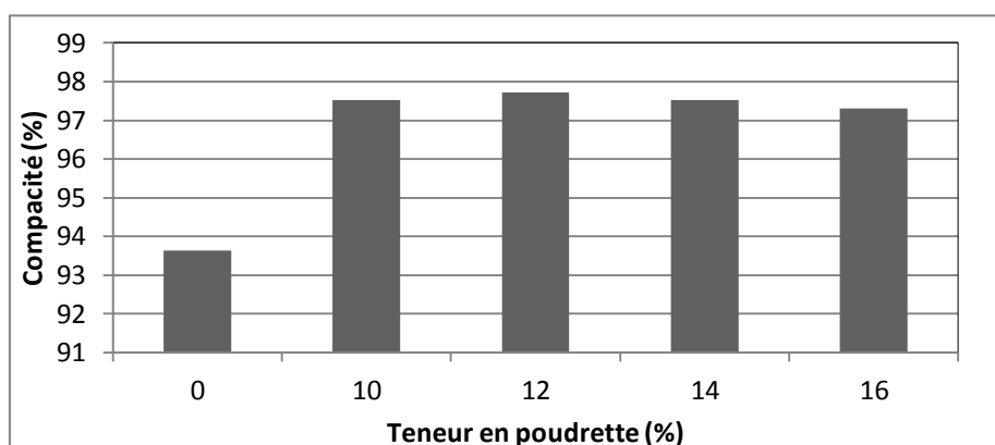
Figure 1. Compacités en fonction de la teneur en déchets « Mode A »
