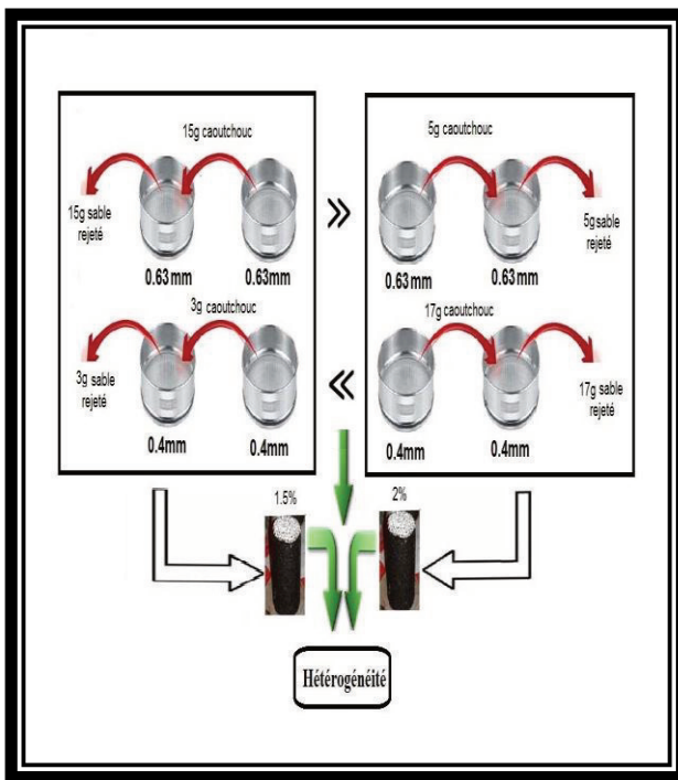
Figure 10. Schéma explicatif d'hétérogénéité en mode B
