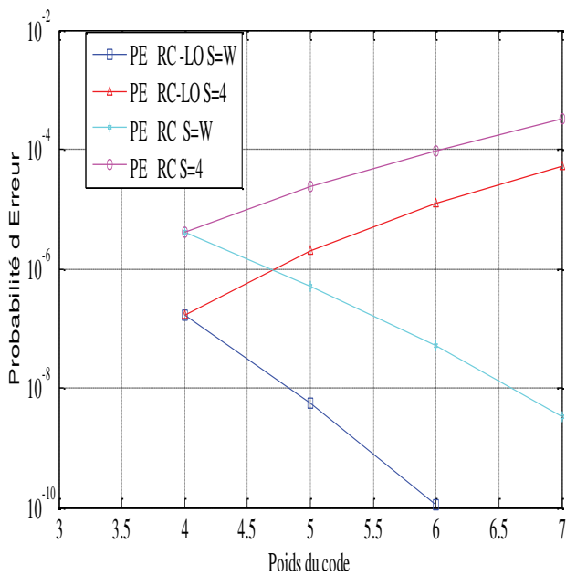
Figure 5. La probabilité d'erreur du RC et du RC-LO en fonction de W pour le code (97,4,1,1), N=8 .
