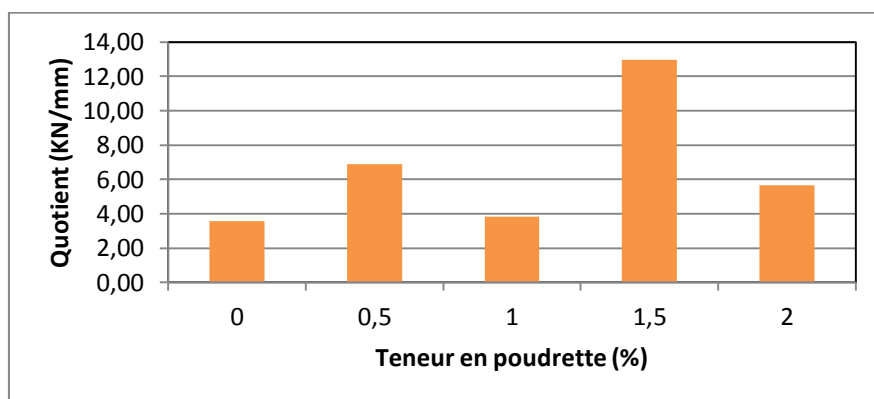
Figure 9. Quotient en fonction de la teneur en déchets « Mode B »
