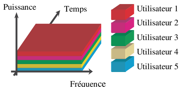
Figure 1. La technique d'accès multiple CDMA.
