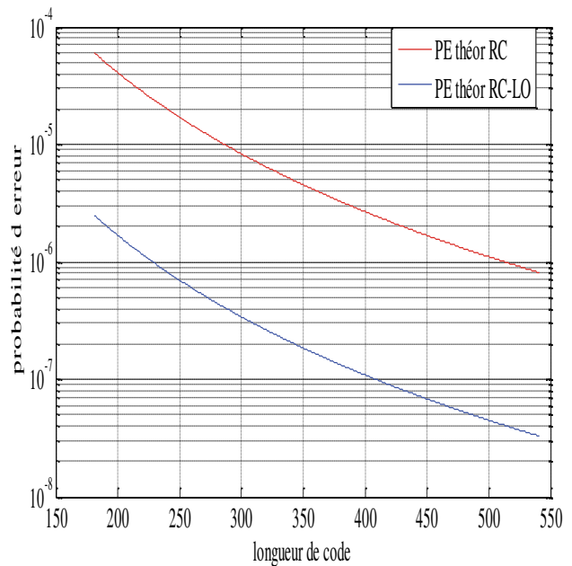
Figure 6. La probabilité d'erreur du RC et du RC-LO en fonction de L pour le code (L,4,1,1), N=8 .
