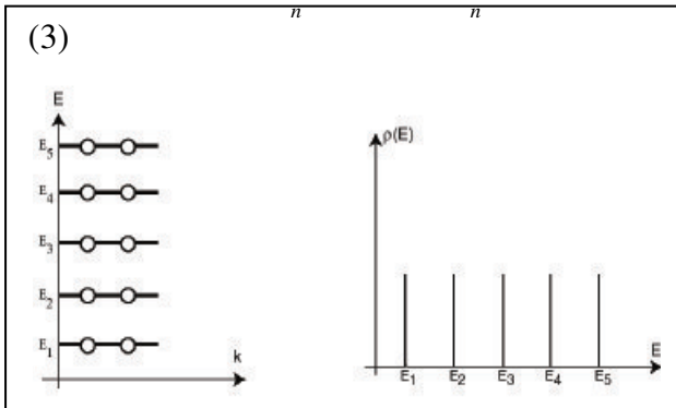
Figure 1. Courbe de dispersion E(k) et densité d'état \rho(E) pour une boîte quantique.
