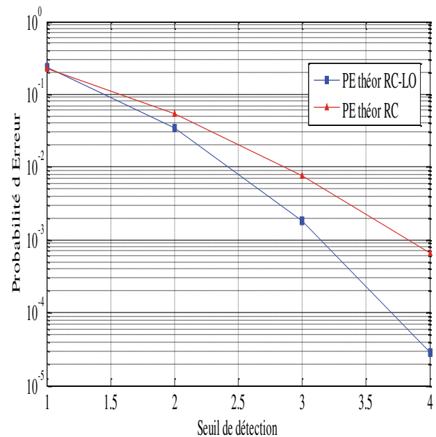
Figure 3. La probabilité d'erreur du RC et RC-LO en fonction en fonction du seuil S pour le code OOC (97,4,1,1), N=8.
