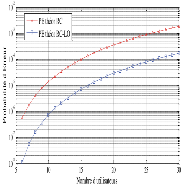
Figure 4. La probabilité d'erreur du RC et du RC-LO en fonction de N pour OOC (97,4,1,1).
