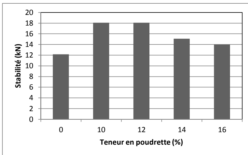
Figure 2. Stabilités en fonction de la teneur en déchets « Mode A »
