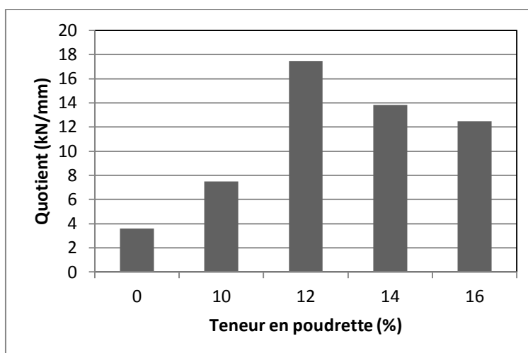
Figure 4. Quotients Marshall en fonction de la teneur en déchets « Mode A »
