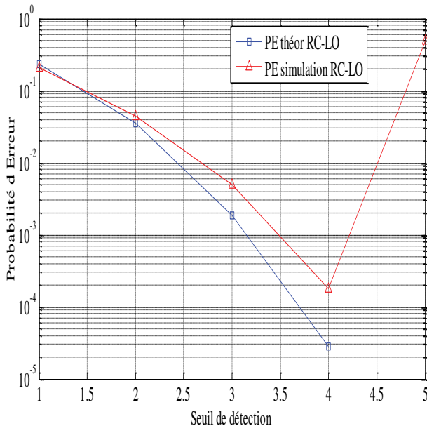
Figure 7. La probabilité d'erreur théorique et simulée correspondant au code OOC (97,4,1,1) avec N=8 pour le récepteur RC-LO.
