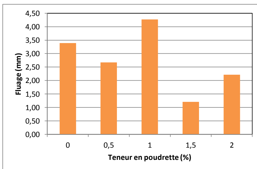
Figure 8. Fluage Marshall en fonction de la teneur en déchets « Mode B »
