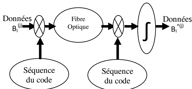
Figure 2. Synoptique d'un système DS-OCDMA.
