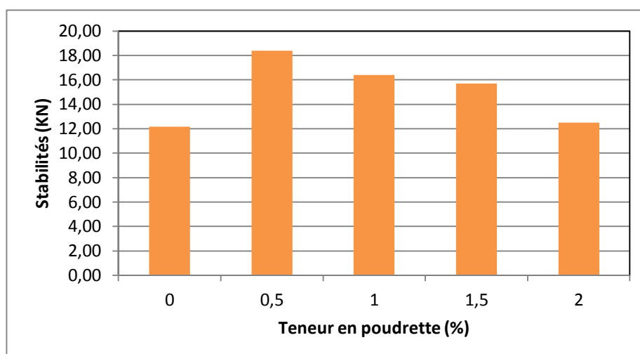
Figure 7. Stabilités en fonction de la teneur en déchets « Mode B »
