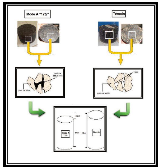
Figure 11. Comparaison entre éprouvette modifiée (12%) et l'éprouvette témoin
