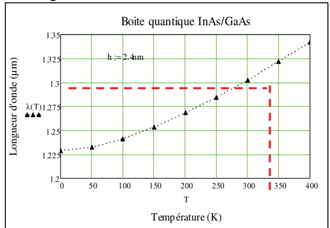
Figure 2. La longueur d'onde en fonction de la température.
