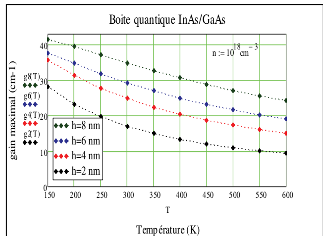
Figure 4. Le gain maximal en fonction de la température pour différentes tailles de boîtes quantiques ( h=8 \text{ nm} , 6 \text{ nm} , 4 \text{ nm} , 2 \text{ nm} ) avec n = 10^{18} \text{ cm}^{-3} .
