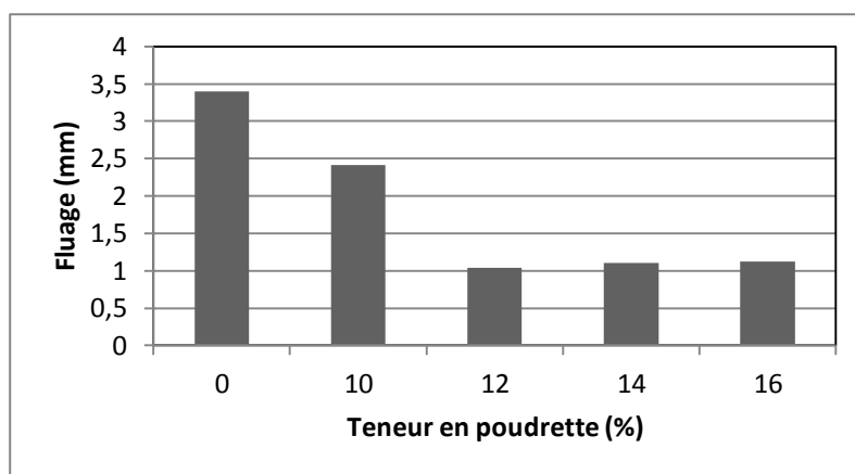
Figure 3. Fluage en fonction de la teneur en déchets « Mode A »
