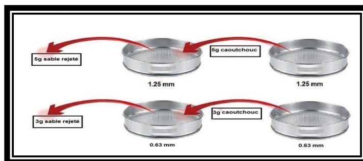
Figure 5. Étapes de compensation par la poudrette (Mode B)
