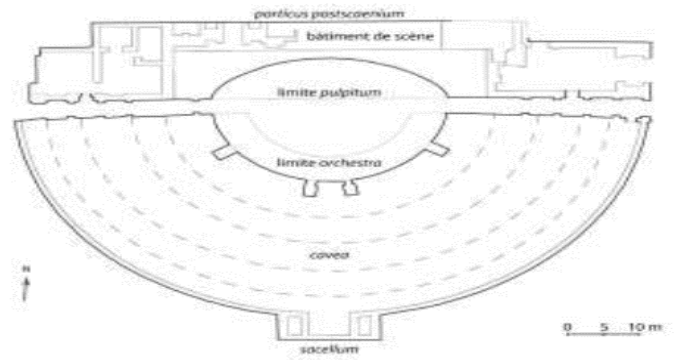
مخطط المسرح نقلا عن : Leveau (Ph.), O.p.Cit, p.35
