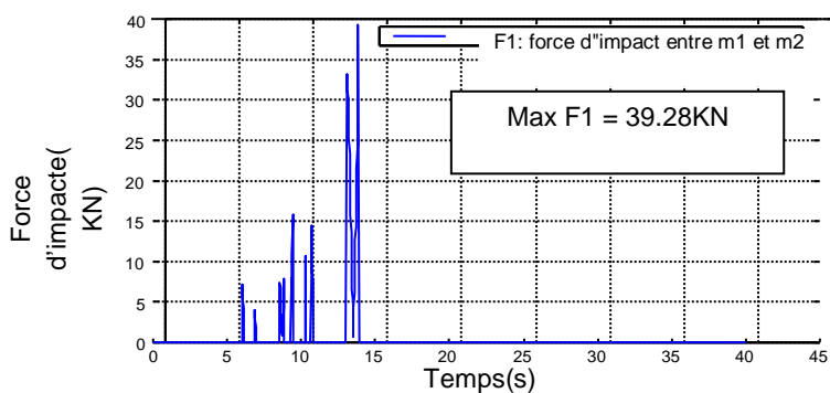
Fig 6.Évolution de la force d'impact entre la 1 ère et la 2 ème structure.
