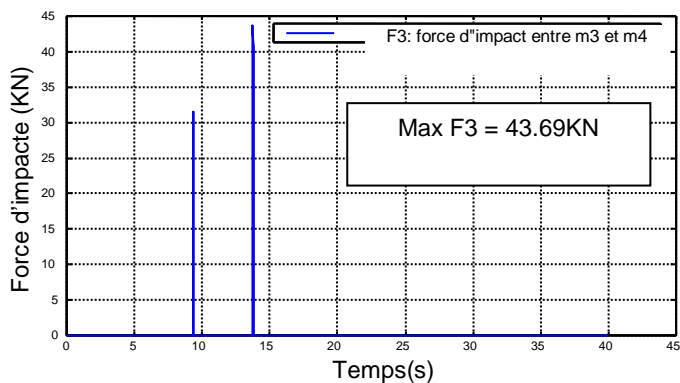
Fig 5.Évolution de la force d'impact entre la 3 ème et la 4 ème structure.
