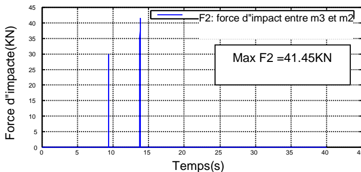
Fig 4.Évolution de la force d'impact entre la 2 ème et la 3 ème
