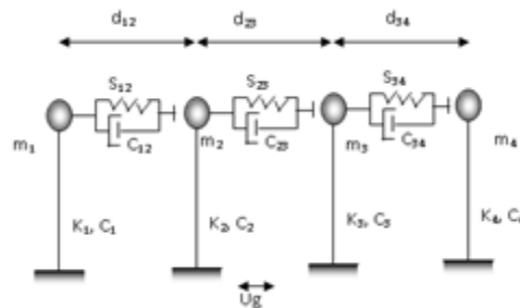
Fig. 1. Modélisation de plusieurs structures adjacentes.
