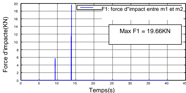
Fig 3. Évolution de la force d'impact entre la 1 ère et la 2 ème
