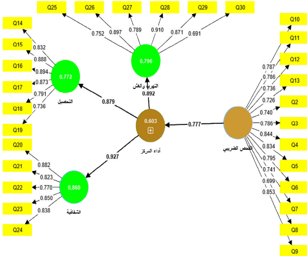
الشكل (01): النموذج البنائي من الدرجة الثانية
