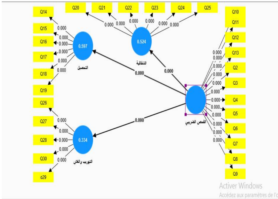
الشكل 02: النموذج البنائي من الدرجة الأولى
