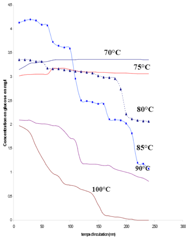
Figure 6 : Courbes de la thermostabilité de l'enzyme.
