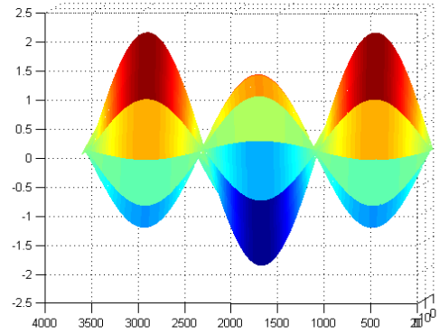
7-c) mode (3,1) ; b=0.1\text{m}
