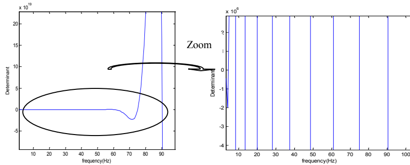
Figure 2 : Evaluation des fréquences libres
