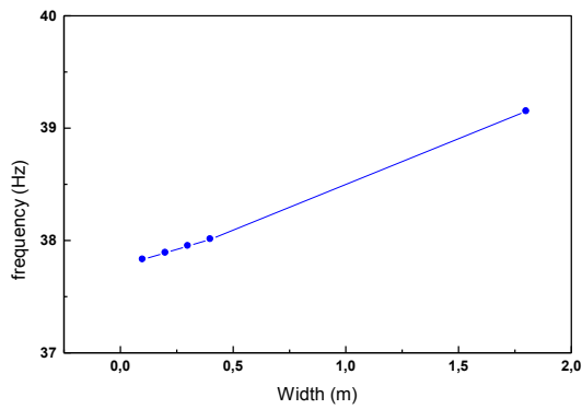
Figure 6 : Evolution des fréquences libres pour le troisième mode.
