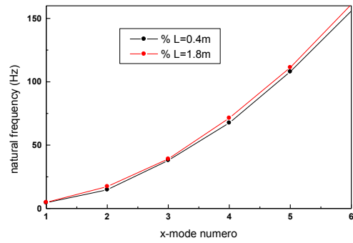
Figure 5 : Evolution des fréquences libres paramétrées par la largeur de la plaque.
