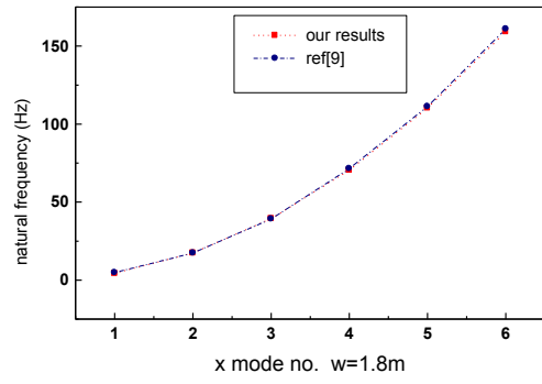
Figure4 : Evolution des fréquences libres avec le mode considéré.
