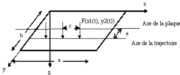
Figure1 : Modèle de la plaque sollicitée par un convoi de charges mobiles.
