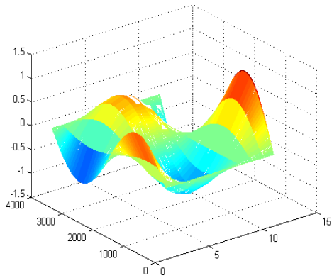
7-b) mode (2,1) ; b=0.1\text{m}
