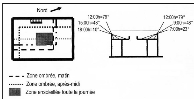
Figure 7: Projection de l'ombre sur la terrasse (23 juillet, 31°Nord).
