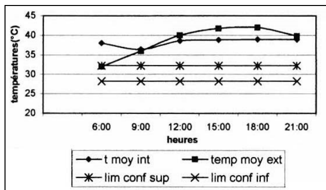
Figure 11: Evaluation de la performance thermique de la chambre (comparaison température intérieure, limites de confort). Période été, Ouargla.
