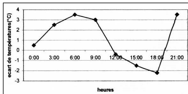
Figure 8: Ecart entre températures tri horaires intérieures et extérieures, chambre- Ouargla, Été 2000.
