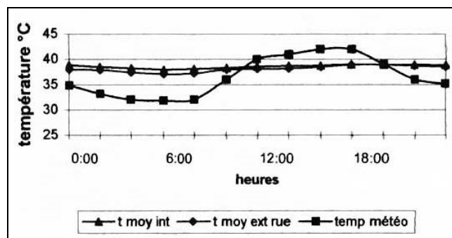
Figure 9a: Comparaison de la température moyenne intérieure - extérieure rue - Météo. Ouargla, Été 2000.
