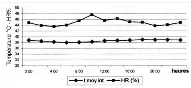
Figure 9b: Variation de température et de l'humidité relative à l'intérieur de la chambre. Ouargla, Été 2000.
