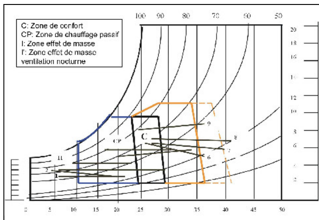
Figure 2: Diagramme psychrométrique de S.-Zockolay appliqué à la ville de Ouargla.
