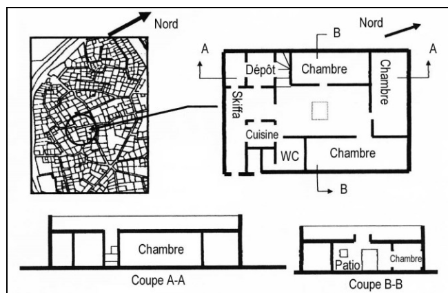
Figure 3: Organisation spatiale, maison traditionnelle Ouargla.
