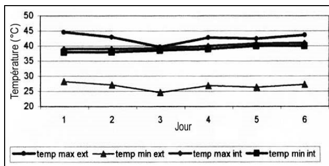
Figure 10: Comparaison des températures maximale et minimale, intérieure et extérieure. Chambre. Ouargla, Été 2000.
