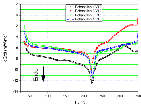
Figure 6 : Courbes de DSC des quatre échantillons obtenues pour V=10 °C/mn.
