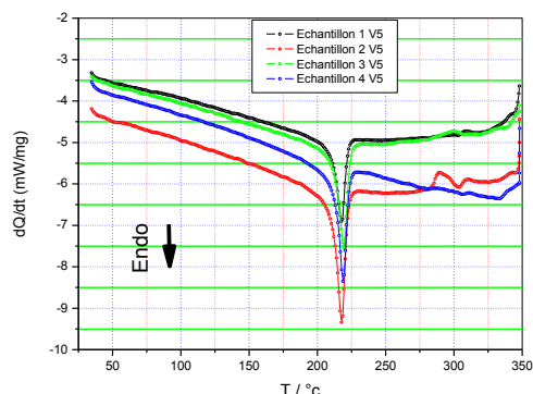
Figure 7 : Courbes de DSC des quatre échantillons obtenues pour V=5 °C/mn.
