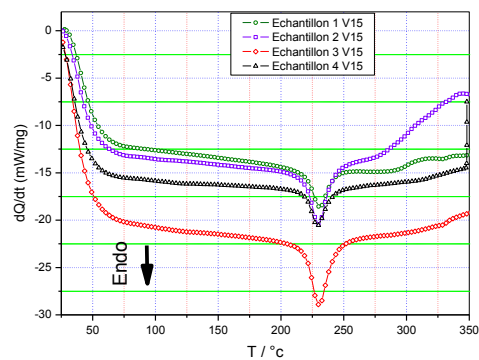
Figure 5 : Courbes de DSC des quatre échantillons obtenues pour V=15 °C/mn.
