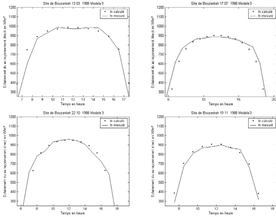
Fig. 3: Comparaison du modèle 3 avec les valeurs mesurées – Site: Bouzaréah (Direct)
