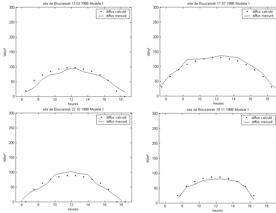
Fig. 9: Comparaison du modèle 1 avec les valeurs mesurées – Site: Bouzaréah (Diffus)
