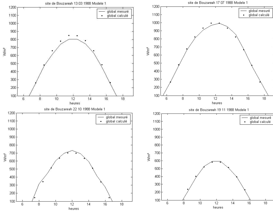
Fig. 17: Comparaison du modèle 1 avec les valeurs mesurées – Site: Bouzaréah (Global)
