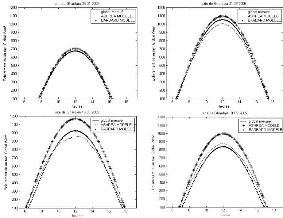
Fig. 24: Comparaison du modèle Ashrae et Barbaros avec les valeurs mesurées Site: Ghardaia (Global)
