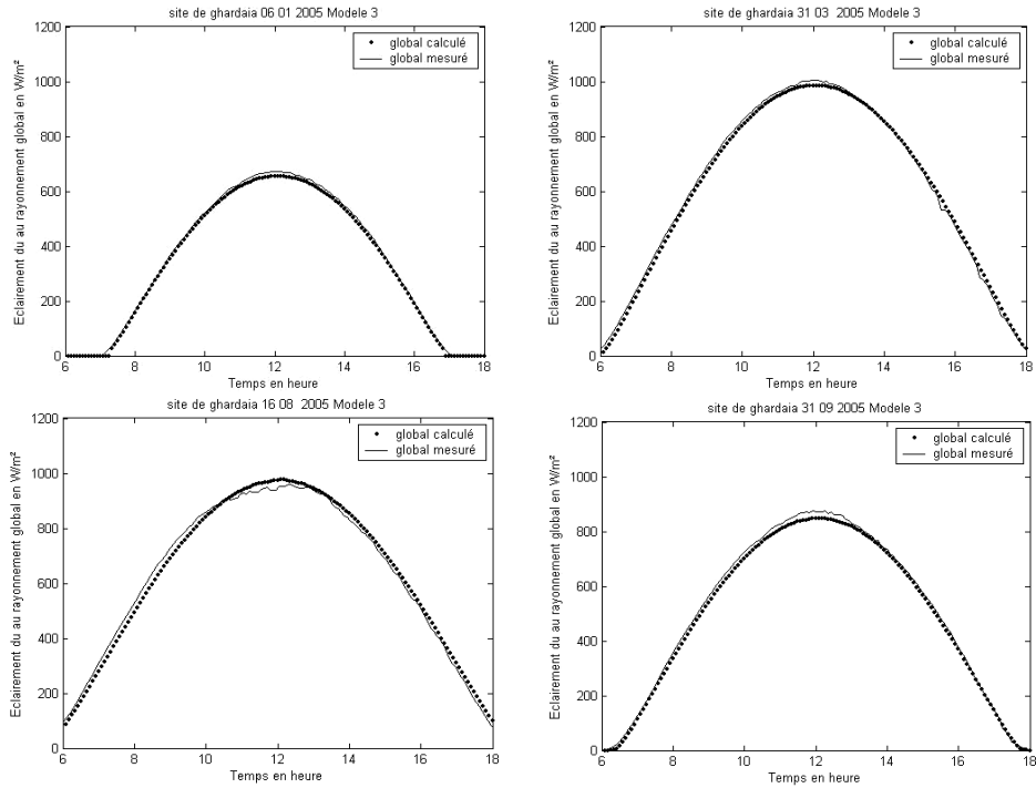
Fig. 23: Comparaison du modèle 1 avec les valeurs mesurées – Site: Ghardaia (Diffus)
