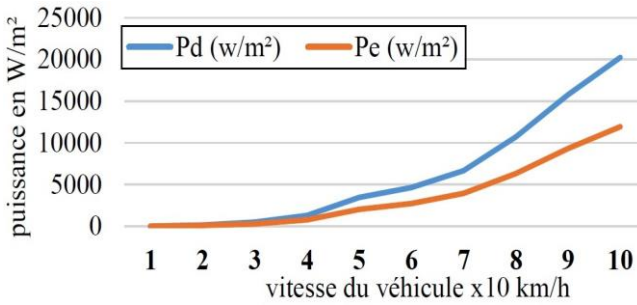
Fig. 5: Variation des puissances disponibles et extractibles en fonction de la vitesse du véhicule
