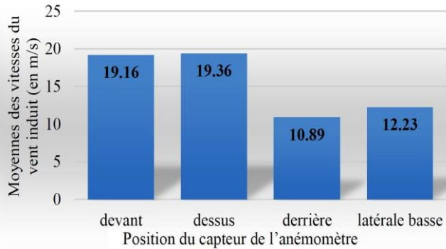
Fig. 3: Comparaison des vitesses moyennes du vent induit à différentes positions du capteur de l'anémomètre
