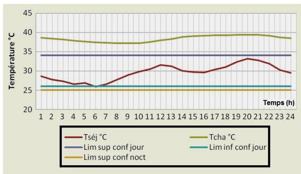
Fig. 11: Comparaison des températures du séjour et la chambre aux limites de confort - Source : Auteur
