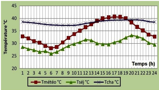
Fig. 8: Variation horaire de la température pendant la période de mesure en été - Source: Auteur
