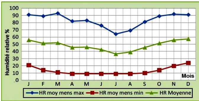
Fig. 2: Variation mensuelle de l'humidité relative de la ville de Biskra
