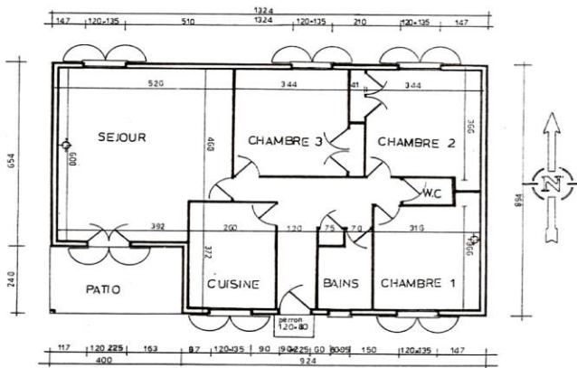
Fig. 5: Vue plan de la maison modèle Source: documents graphiques ENICAB
