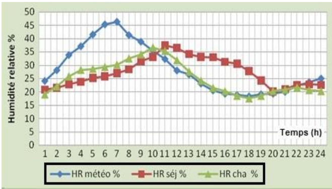
Fig. 9: Variation horaire de l'humidité relative pendant la période de mesure en été - Source: Auteur
