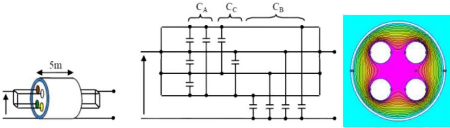
Fig. 8: Essai MC 4 BCO, Schéma de simulation et la répartition du champ magnétique dans le câble
