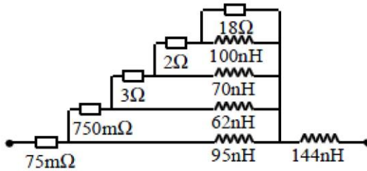
Fig. 9: Réseau RL en échelle
