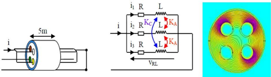
Fig. 5: Essai MC 3 BCC, Schéma de simulation et la répartition du champ magnétique dans le câble
