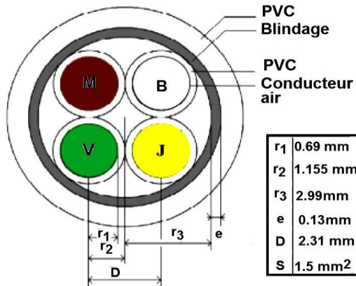
Fig. 1: Câble dissymétrique blindé composé de 04 conducteurs
