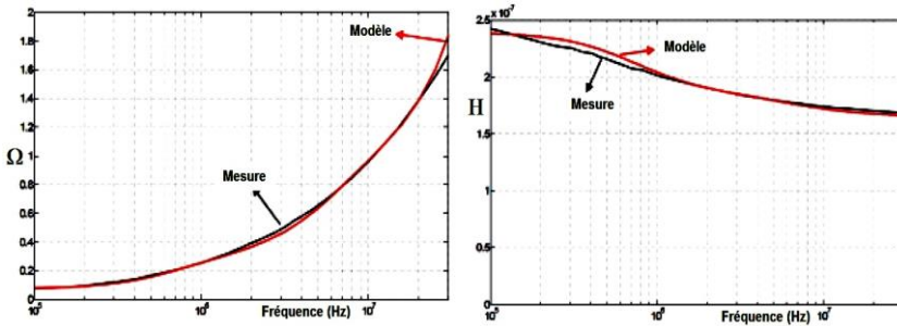
Fig. 10: Evolution de R et L en fonction de la fréquence
