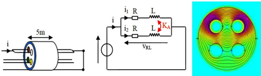
Fig. 3: Essai MC 2 BCC, Schéma de simulation et la répartition du champ magnétique dans le câble
