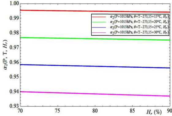
Fig. 6: Evolution de \alpha_2 en fonction de H à P et T constante
