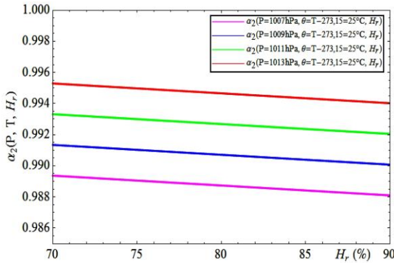
Fig. 7: Evolution de \alpha_2 en fonction de H à P et T constante
