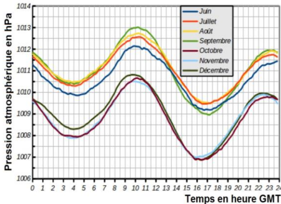
Fig. 2: Evolution de la pression atmosphérique des sept derniers mois de 2011
