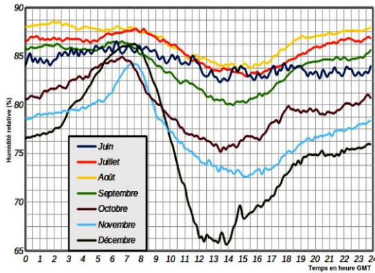
Fig. 1: Evolution de l'humidité relative des sept derniers mois de 2011
