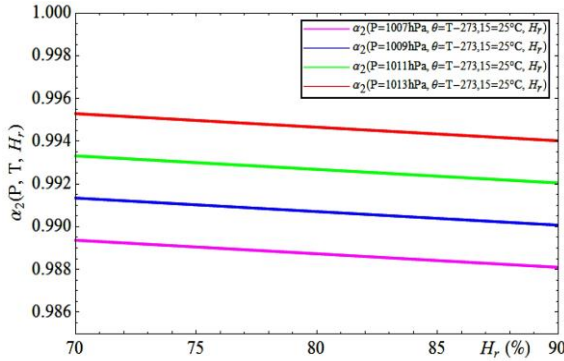
Fig. 6: Evolution de \alpha_2 en fonction de H à P et T constante
