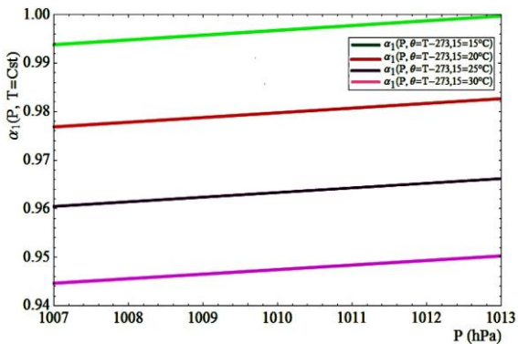
Fig. 5: Evolution de \alpha_1 en fonction de P à T constante
