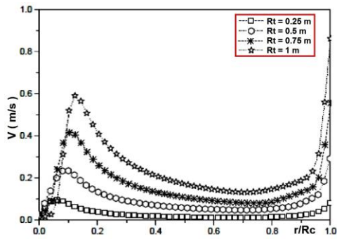
Fig. 9: Influence du diamètre de la tour sur le profil de vitesse le long du collecteur pour \Delta T = 10^\circ C à X = 0.025 m
