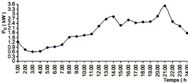
Fig. 10: Consommation journalière d'une station GSM [16]
