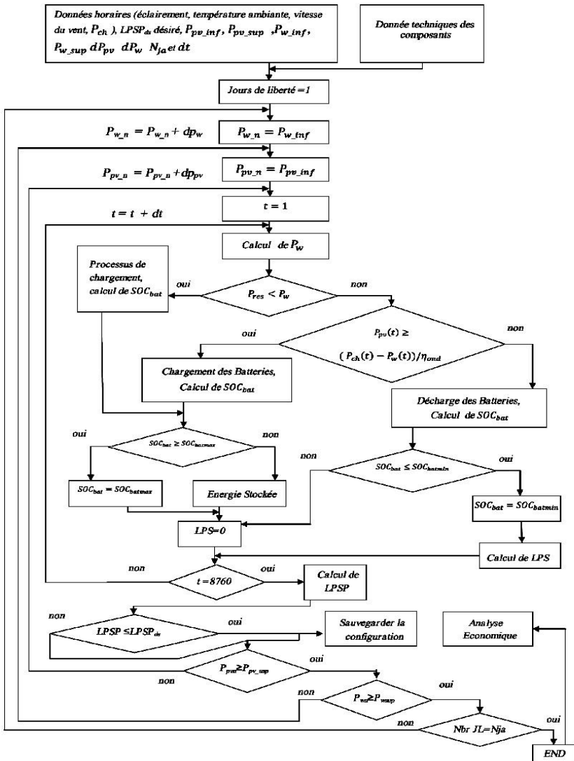
Fig. 3: Organigramme global de l’algorithme de dimensionnement
