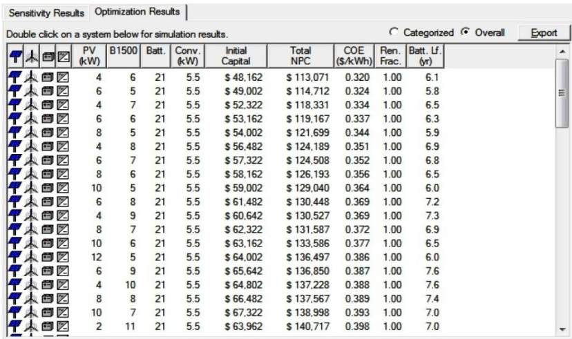
Fig. 17: Résultats de dimensionnement par le logiciel Homer
