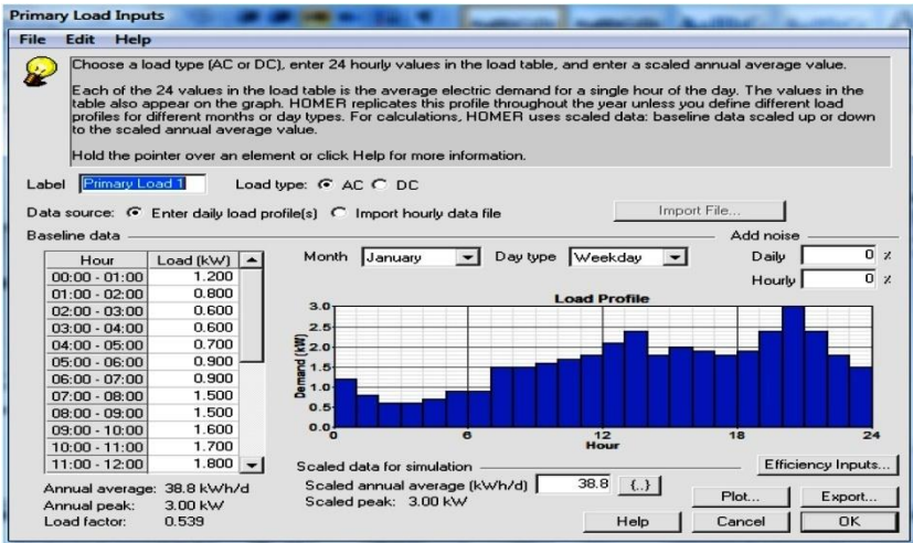
Fig. 15: Profil de charge de la station GSM
