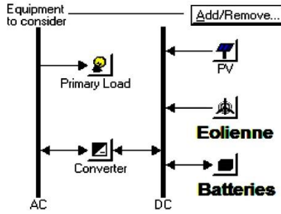
Fig. 14: Configuration de l’installation à dimensionner
