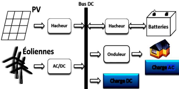
Fig. 1: Architecture du système étudié
