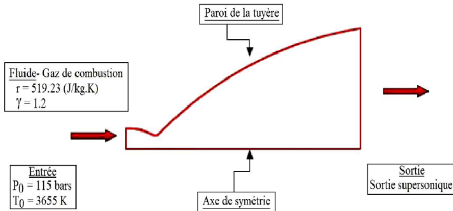
Fig. 1: Domaine de calcul et conditions aux limites
