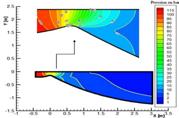
Fig. 6: Distribution de la pression statique en bars
