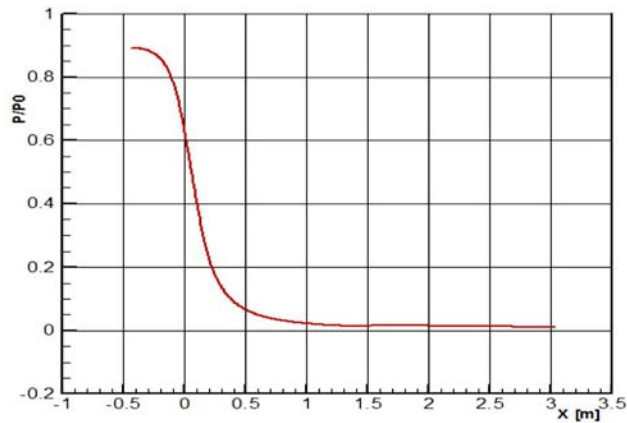
Fig. 7: Profil de pression statique axiale adimensionnelle
