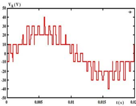
Fig. 5: Tension de sortie de la première phase V_A et son analyse spectrale
