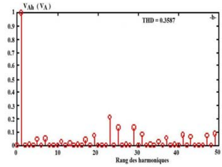
Fig. 5: Tension de sortie de la première phase V_A et son analyse spectrale
