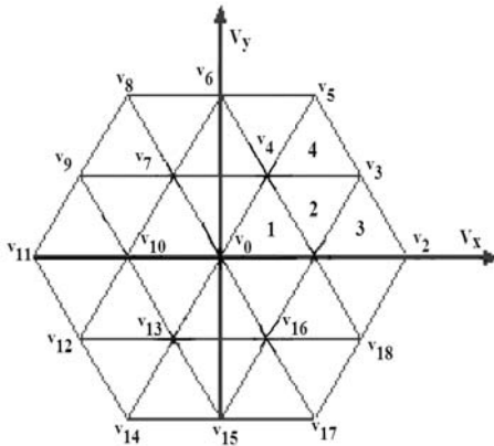
Fig. 2: Diagramme vectoriel de l'onduleur
