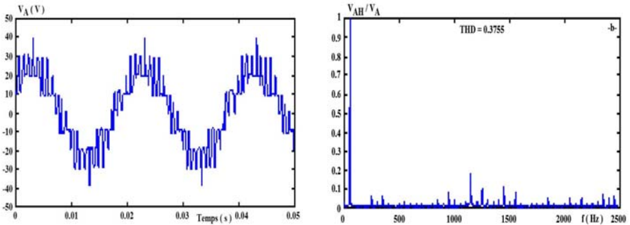
Fig. 12: Tension de sortie de la première phase V_A et son analyse spectrale
