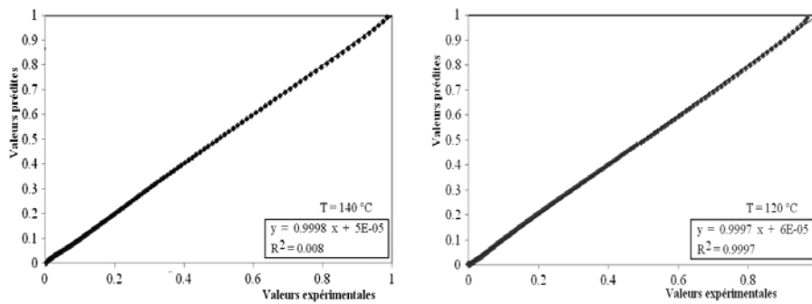
Fig. 6: Comparaison entre les valeurs expérimentales et les valeurs prédites par le modèle polynomial du 4 ème degré pour 'Boue B' et pour diverses températures de séchage (Trait continu : valeur prédite, Point : valeur expérimentale)
