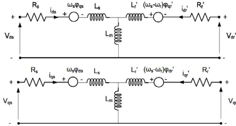
Fig. 8: Schéma équivalent de la machine asynchrone selon l'axe 'd' et l'axe 'q'
