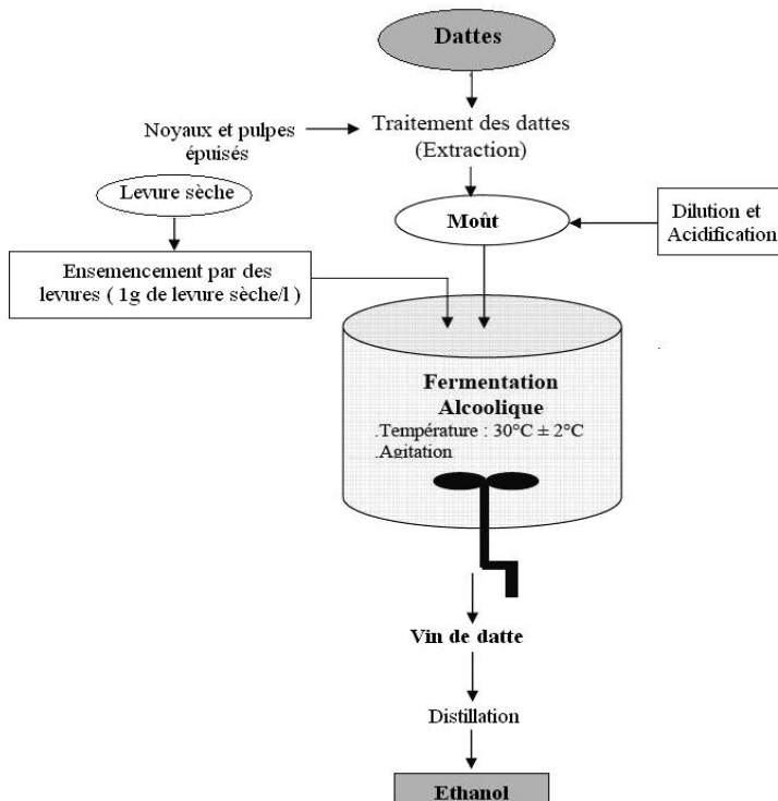
Fig. 5: Diagramme de déroulement de la fermentation alcoolique
