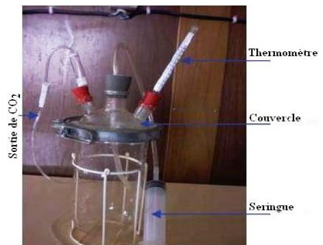
Vue du bioréacteur
