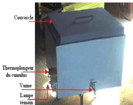
Vue du bain marie
