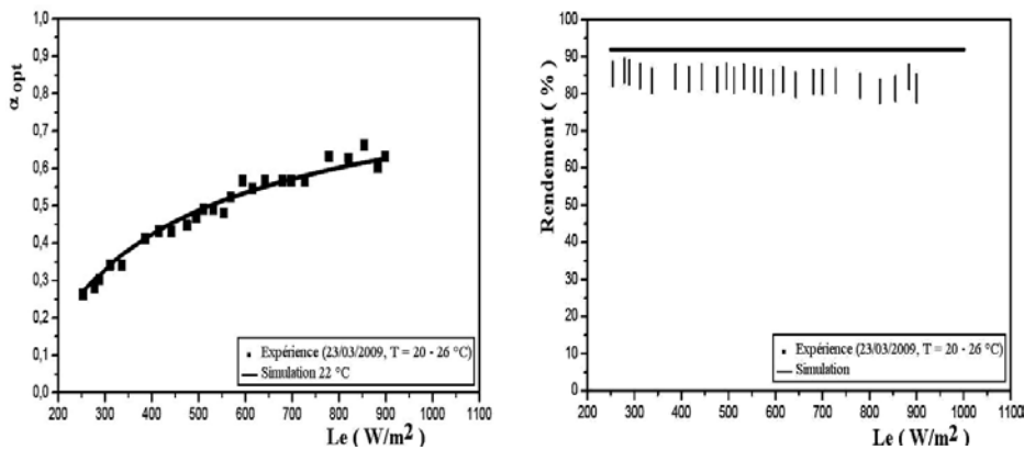
Fig. 8: Rapport cyclique et rendement optimaux expérimentaux (■, |) et simulés dans Pspice (—). 23/03/2009. T: 22 - 25°C.
