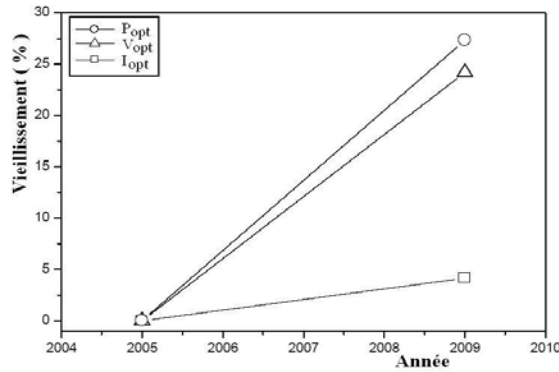
Fig. 15: Dégradation de la tension V_{opt} , du courant I_{opt} et puissance P_{opt} optimaux en fonction des années
