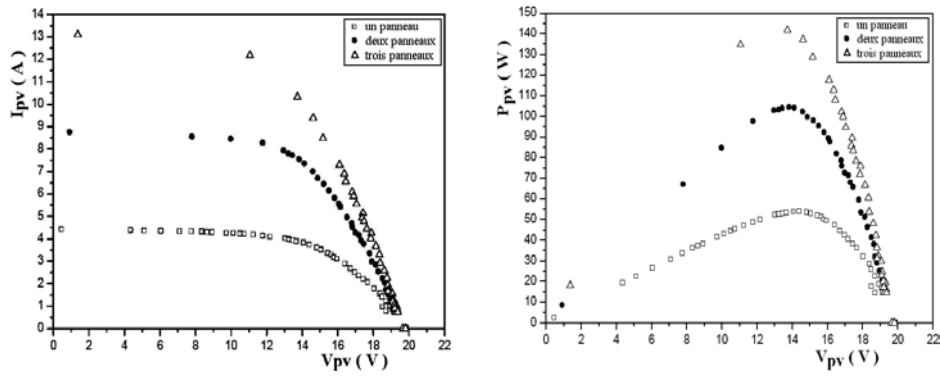
Fig. 9: Caractéristiques courant-tension et puissance-tension expérimentales de un, deux et trois modules montés en parallèle. 01/04/2009, T: 22 – 25 °C, L_e = 917 \text{ W/m}^2
