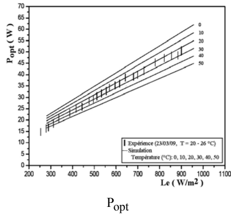
Fig. 7: Grandeurs électriques optimales ( V_{opt} , I_{opt} et P_{opt} ) expérimentales (|) et simulées dans Pspice (—). 23/03/2009, T: 22-25°C
