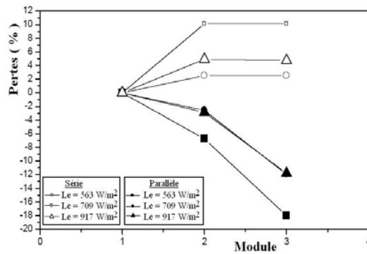
Fig. 13: Pertes (amélioration) de la puissance optimale d'un module, lors l'association des modules en parallèle (série) en fonction de l'éclairement. 03/2009, T: 22 – 25 °C
