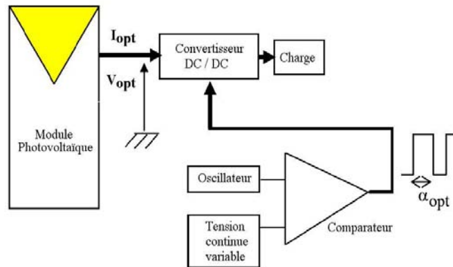
Fig. 6: Régulation manuelle de la puissance fournie par le module photovoltaïque
