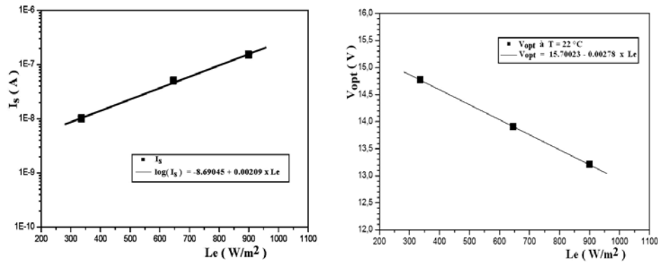
Fig. 5: Variation du courant de saturation ( I_S ) et de la tension optimale ( V_{opt} ) en fonction de l'éclairement. 23/03/2009, T: 22 – 25 °C.
