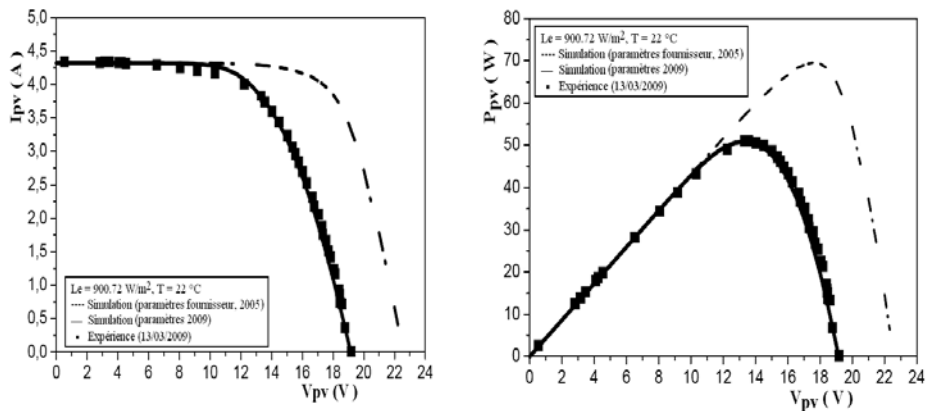
Fig. 14: Caractéristiques courant-tension et puissance-tension expérimentales et simulées en tenant compte des caractéristiques expérimentales et celles fournies par le fabricant
