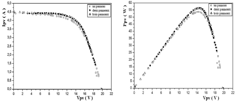
Fig. 12: Caractéristiques courant-tension et puissance-tension expérimentales d'un module, déduites des caractéristiques de la figure 10 (01/04/2009, T: 22 – 25 °C, Le = 917 \text{ W/m}^2 )
