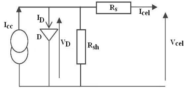
Fig. 1: Schéma électrique d'une cellule photovoltaïque
