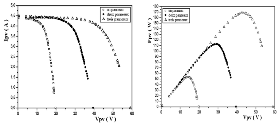
Fig. 10: Caractéristiques courant-tension et puissance-tension expérimentales de un, deux et trois modules montés en série. 01/04/2009, T: 22 – 25 °C, L_e = 917 \text{ W/m}^2
