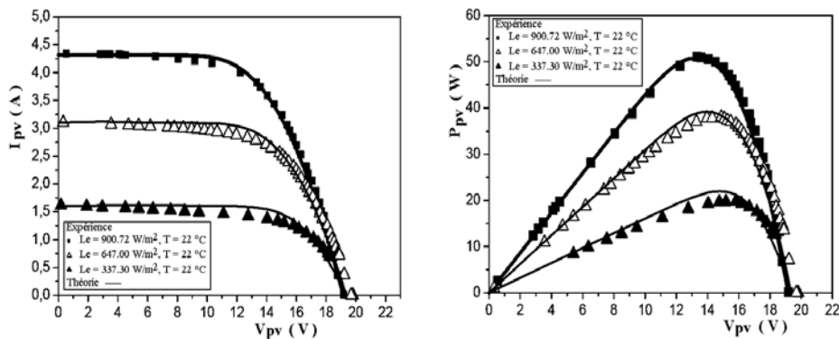
Fig. 4: Caractéristiques courant-tension et puissance-tension expérimentales (■, △, ▲) et simulées dans Pspice (—). 23/03/2009, T: 22 – 25 °C
