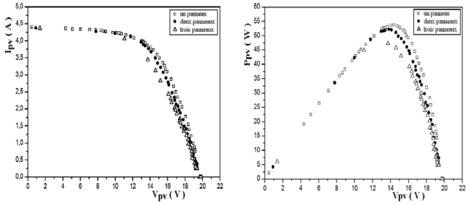
Fig. 11: Caractéristiques courant-tension et puissance-tension expérimentales d'un module, déduites des caractéristiques de la figure 9 (01/04/2009, T: 22 – 25 °C, Le = 917 \text{ W/m}^2 )
