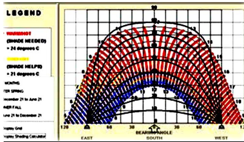
Fig. 5: Sun shading chart, tiré de 'CC04'
