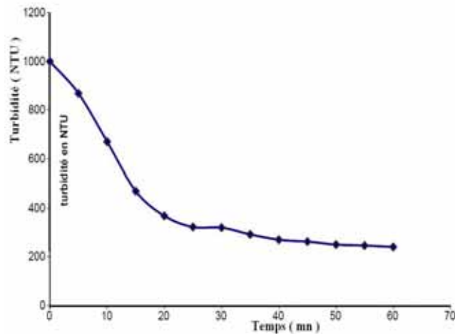
Fig. 2: Suivi de la turbidité en fonction du temps de décantation en dehors de tout traitement
