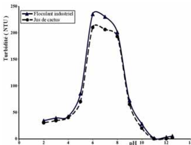
Fig. 3: Variation de la turbidité en fonction de pH Optimisation de pH
