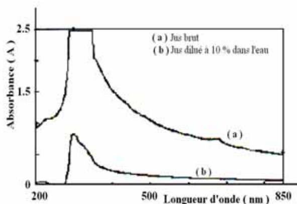
Fig. 1: Spectre d'absorbance UV de jus de cactus vers 300 nm. (a) Jus brut, (b) Jus dilué à 10 % dans l'eau
