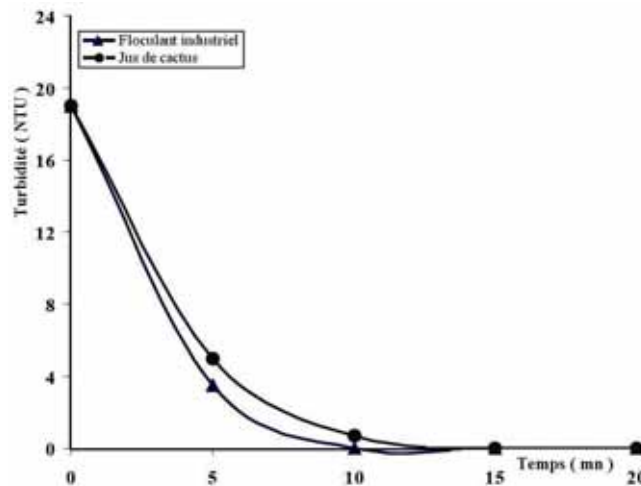
Fig. 5: Variation de la turbidité en fonction du temps de décantation à pH=11 Optimisation du temps de décantation
