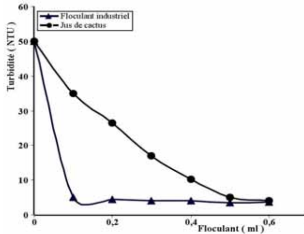
Fig. 4: Variation de la turbidité en fonction du volume de flocculants (ml) Optimisation de la concentration de floculation
