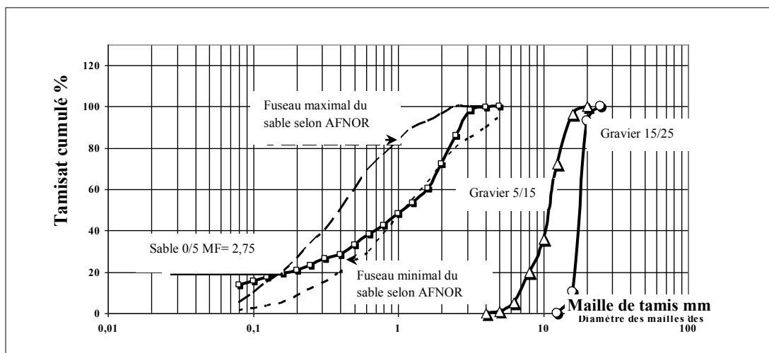
Figure.1 : Courbe granulométrique des granulats utilisés pour la confection des bétons armés (A et B) dosés à 350 kg/m 3 .
