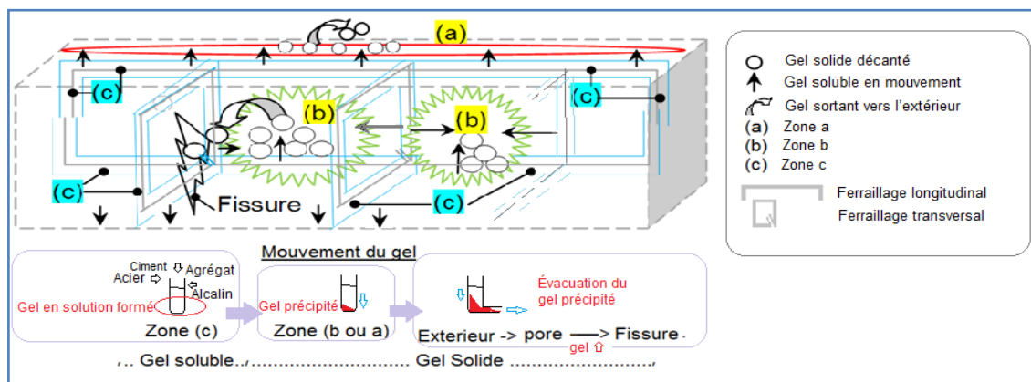
Figure.17 : États du gel de l'AAR formé et son mouvement interne dans une poutre 120 x 20 x 15 cm en béton alcali réactif (B) durant 6 mois, conservé dans des conditions favorables à l'AAR.
