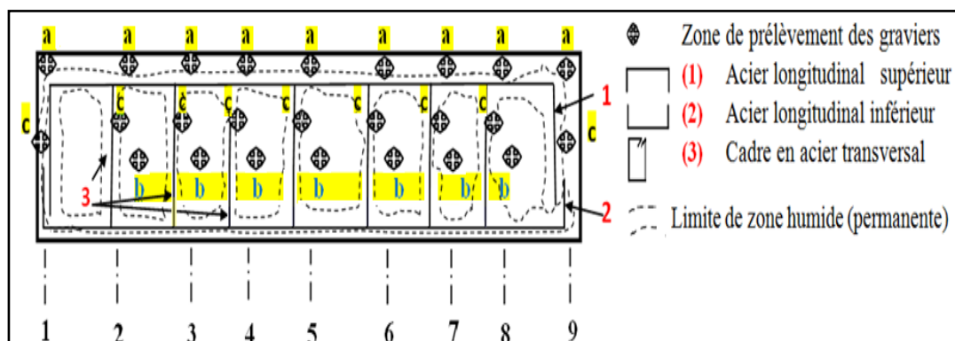
Figure.3 : Prélèvement des échantillons de graviers dans les poutres en béton armé 120x20x15 cm.
