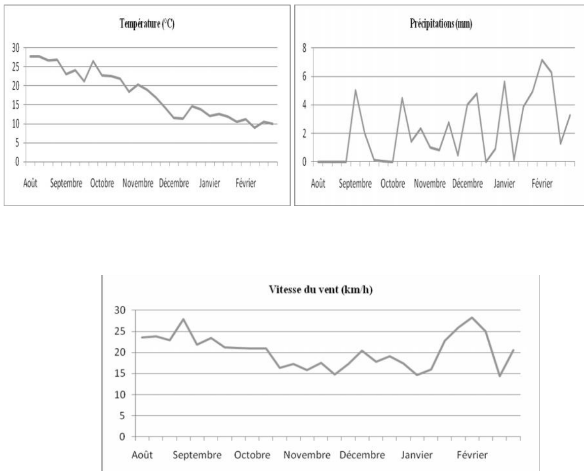
Figure 5 : Variations hebdomadaires des facteurs météorologiques durant la période d'étude dans la région d'Annaba ( www.freemeteo.com ).
