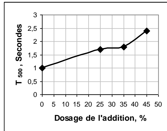
Figure 7 Evolution du temps d’écoulement ( T_{500} ) en fonction du taux de l’addition
