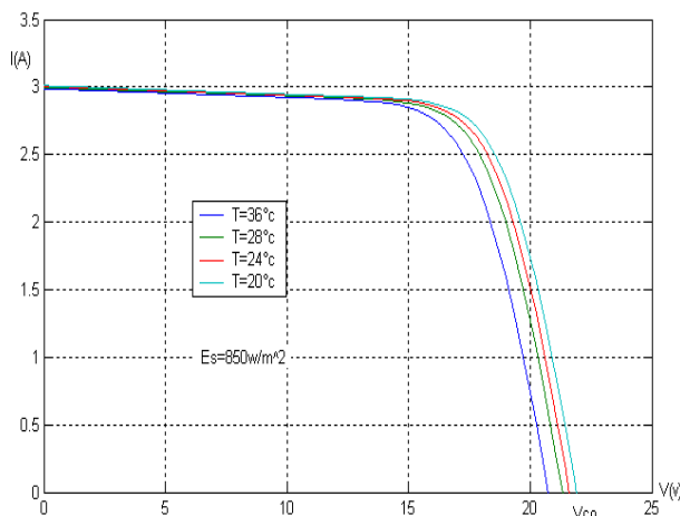
Figure 12. Influence de la température sur la caractéristique I (V).
