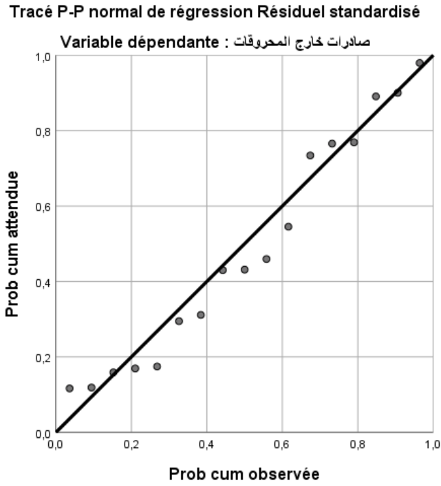
الشكل رقم (1): شكل توزيع البواقي
