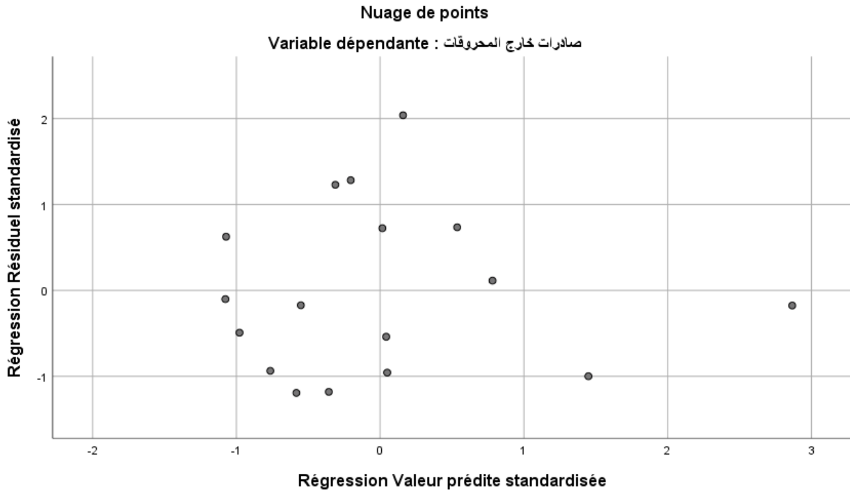
الشكل رقم (3): شكل الانتشار لليواقى مع القيم المتوقعة
