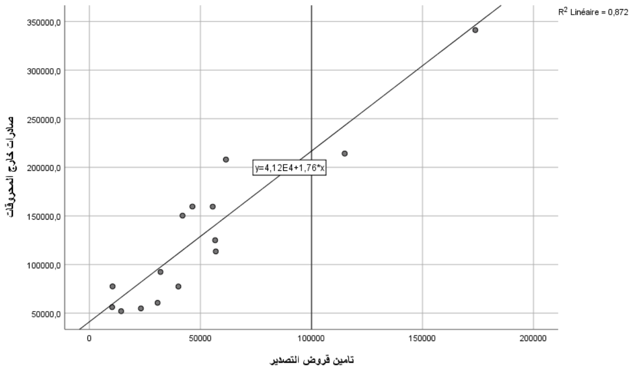
الشكل رقم (4): لوحة الانتشار " معادلة خط الانحدار للنموذج الخطى البسيط "
