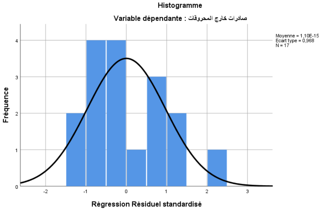
الشكل رقم (2): التوزيع الطبيعي لدراسة
