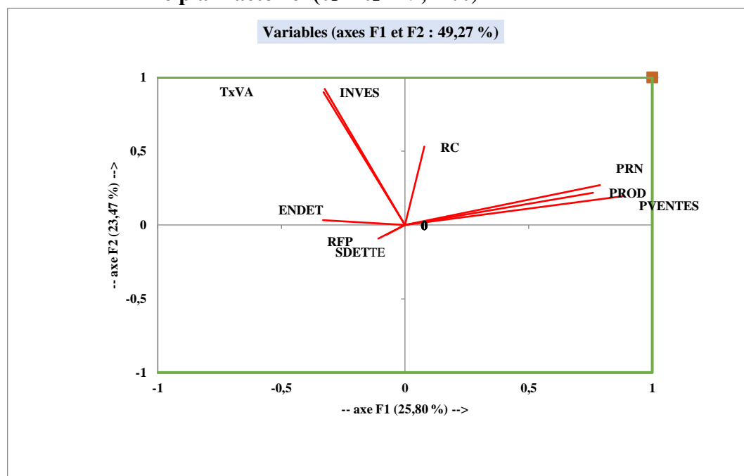
Figure N° 2: Représentation des points variables j de N(j) dans l'espace factoriel (1, 2) « Le plan factoriel ( \tau_1 + \tau_2 = 49,27\% ) »
