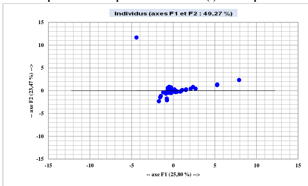
Figure N° 3: Représentation des points individus i de N(I) dans l'espace factoriel (1, 2)
