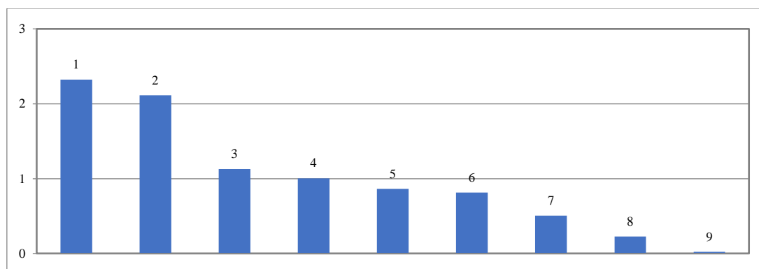
Figure N° 1: Valeurs propres de la matrice des corrélations.
