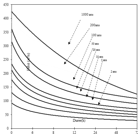
Fig. 4 Modèle QDF (Sidi Bel Abbès).
