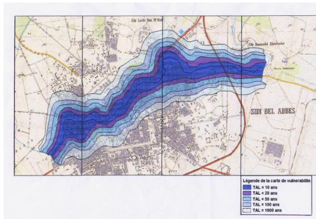
Fig. 5 Aspect de l'aléa
