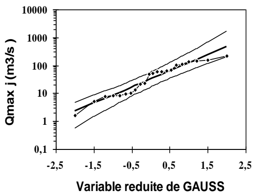
Fig. 2 Ajustement des débits max journaliers à loi log-normale : Station de Sidi Bel Abbès
