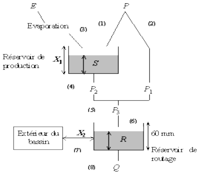
Fig.1. Structure du modèle GR2M
