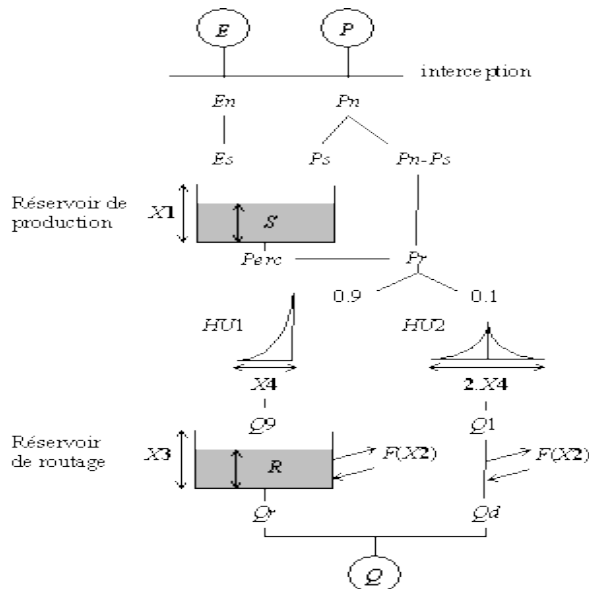
Fig.2. Structure du modèle GR4J
