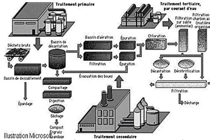
الصورة رقم: متعلقة رسم تخطيطي لمختلف مراحل تصفية المياه المستعملة. [9]
