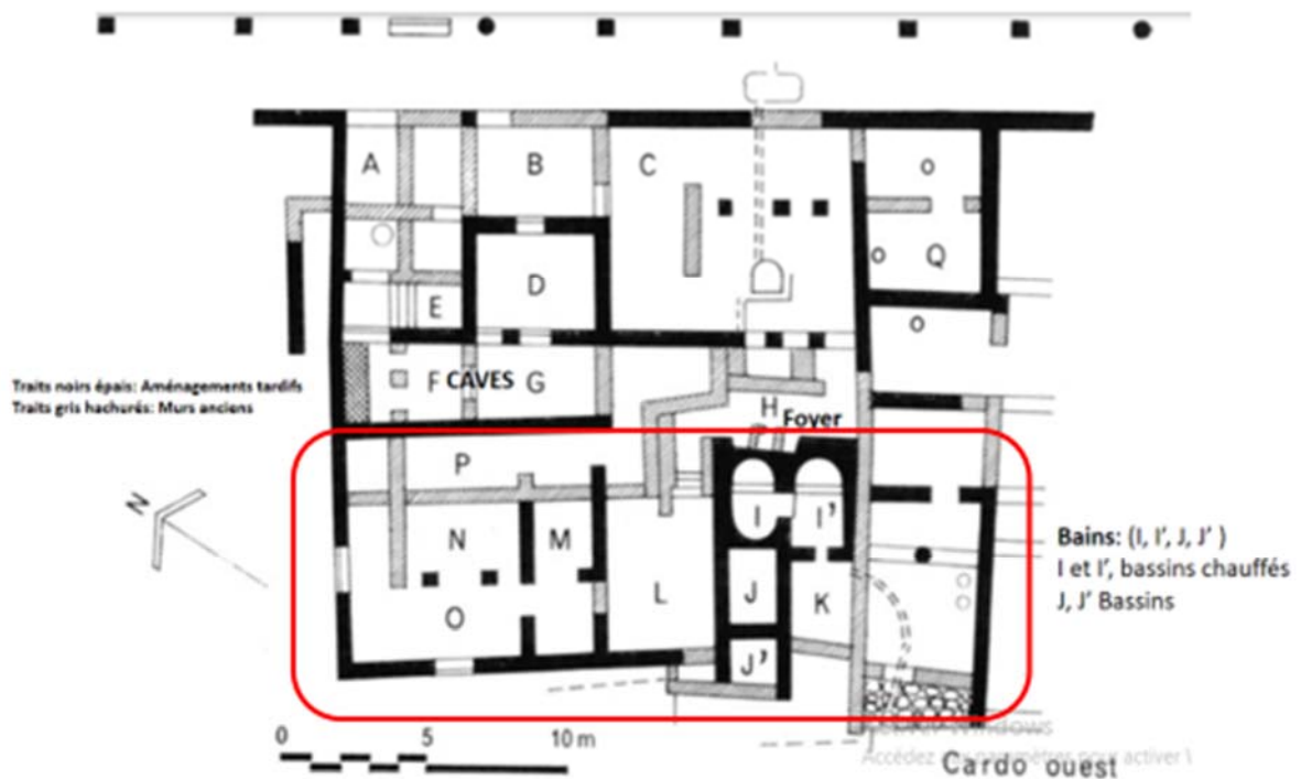
Plan 6 : Maison aux petits bassins à Djemila. En rouge l'atelier
