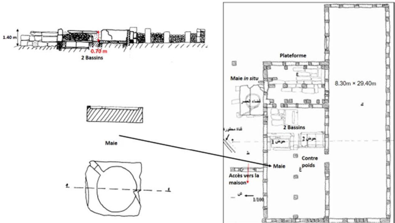
Fig. 1 : Huilerie de la maison au Sud de la porte de Lambèse à Timgad. (Plan et coupe)
