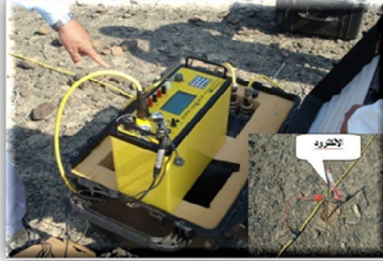
الصورة رقم 01: صورة توضح جهاز المقاومة الكهربائية - المصدر موقع البيان
