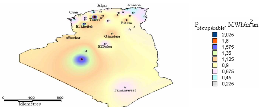
Figure n° 04 : Atlas de la Puissance énergétique Récupérable à 50 m
