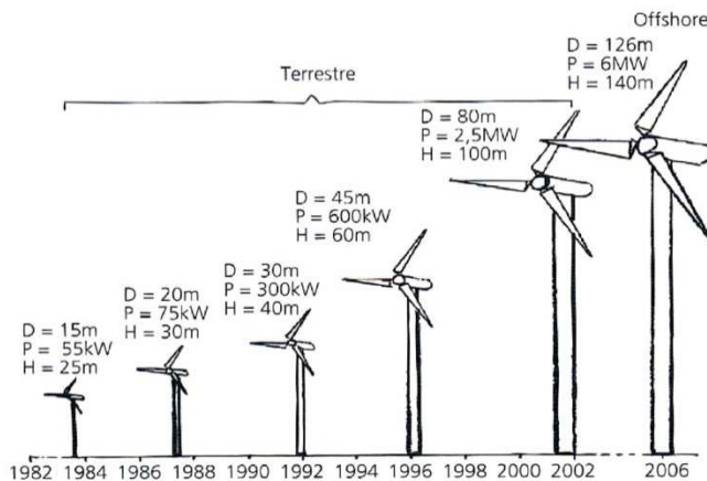
Figure n°01 : Evolution des caractéristiques d'une éolienne depuis 1984
