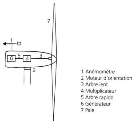
Figure n°03 : Schéma de principe d'une nacelle d'éolienne
