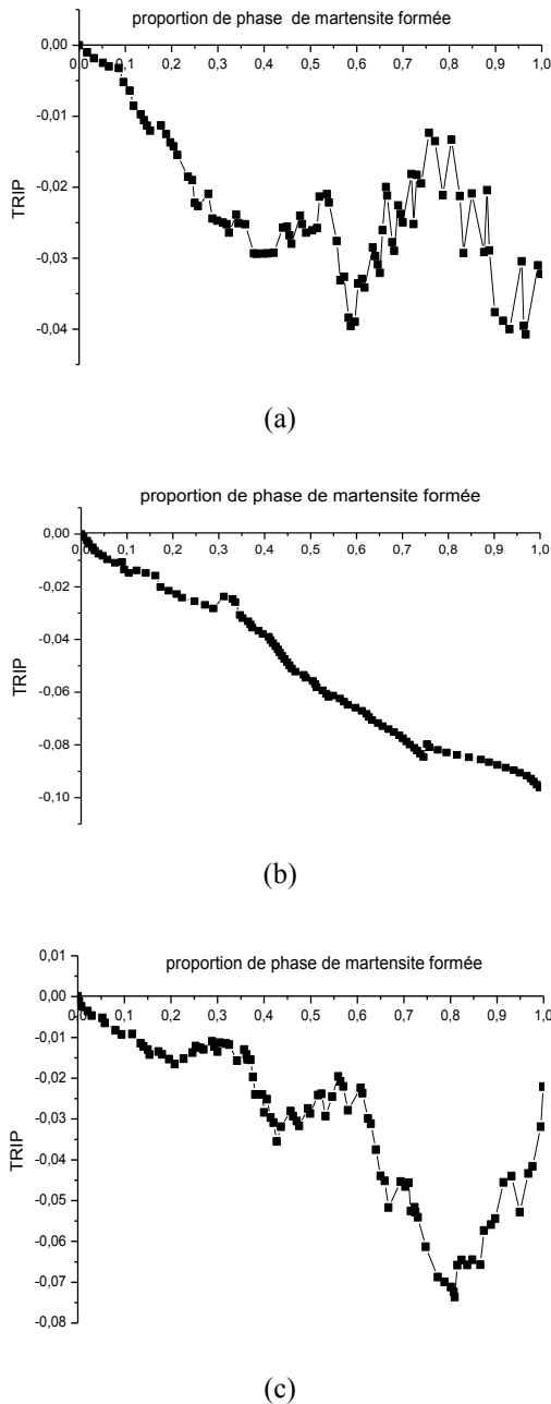
Figure 5 : Evolution de la TRIP sous une contrainte de compression avec la première direction de cisaillement : a) critère de la force mécanique de cisaillement (FMC) b) force moyenne (FMMmoy) c) énergie de déformation élastique locale (EDEL)
