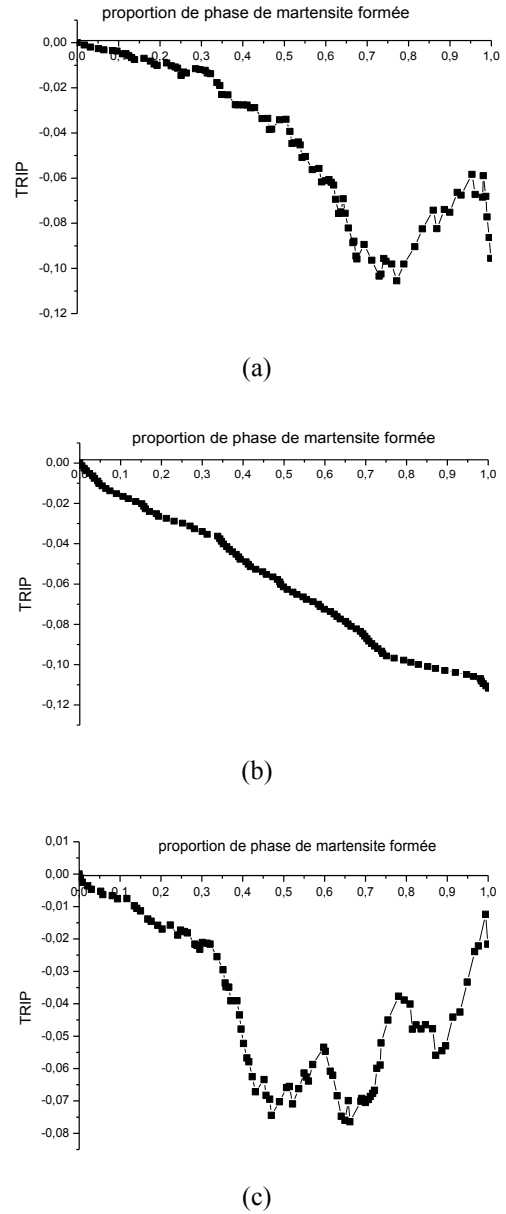
Figure 6 : Evolution de la TRIP sous une contrainte de compression avec la deuxième direction de cisaillement : a) critère de la force mécanique de cisaillement (FMC) b) force moyenne (FMMmoy) c) énergie de déformation élastique locale (EDEL)
