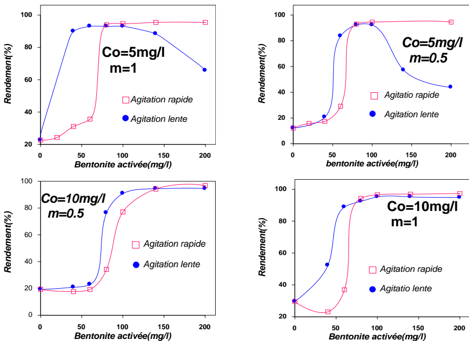
Figure 3 : Elimination de l'acide humique en eau distillée en présence du sulfate d'aluminium et la bentonite activée combinés pour des temps d'introduction différents.
