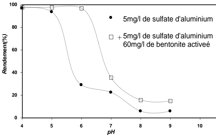
Figure 4 : Effet du pH sur l'élimination de l'acide humique (5mg/l) en eau distillée
