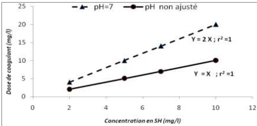
Figure 2 : Relation entre les doses optima en coagulant et les teneurs initiales en acide humique en eau distillée (pH non ajusté ; pH=7)
