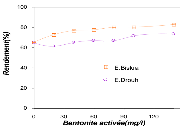
Figure 5 : Elimination de l'acide humique (5mg/l) en eaux minéralisées par combinaison sulfate d'aluminium/bentonite activée ; Dose du sulfate d'aluminium=10mg/l
