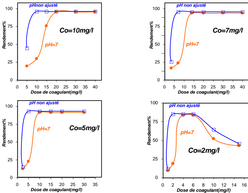
Figure 1 : Evolution des rendements d'élimination de l'acide humique en eau distillée en fonction de la dose de coagulant (pH=7 ; pH non ajusté)
