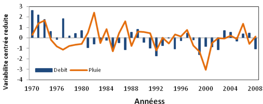
Figure 7 : Sensibilité hydrologique de la Marahoué aux variations annuelles de la pluie. : Cas de la station de Bouaflé (1970-2008)
