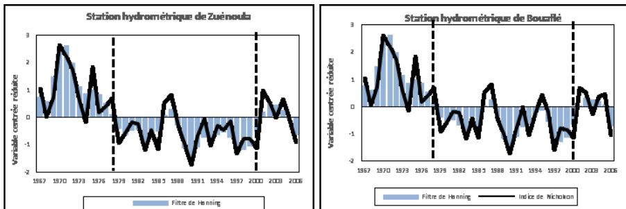
Figure 6 : Variation des modules annuels des débits de la Marahoué à Zuénoula et Bouaflé (1967-2008)
