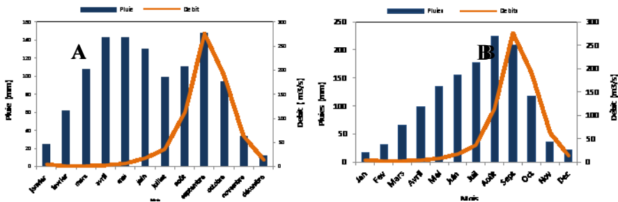
Figure 8 : Variations moyennes mensuelles des écoulements à Bouaflé en fonction de la pluviométrie à Boundiali A) et Bouaflé B), entre 1970-2008
