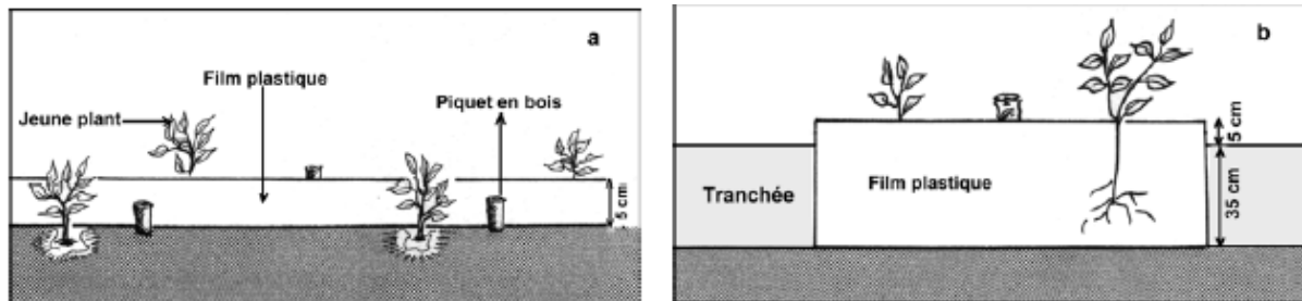
Fig.1 : Installation du film plastique polyéthylène en fixation mécanique des dunes a)- Vue de près ; b)- Coupe longitudinale d'une tranchée
